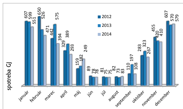
Graf č. 14: Porovnanie Vyrobených GJ pre potreby Výroby tepla a teplej úžitkovej vody v hlavnej budove 2012–2014
