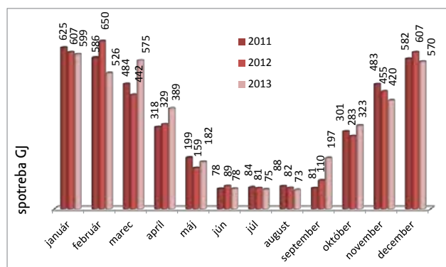
Graf č. 12: Porovnanie Vyrobených GJ pre potreby Výroby tepla a teplej úžitkovej vody v hlavnej budove 2011–2013
