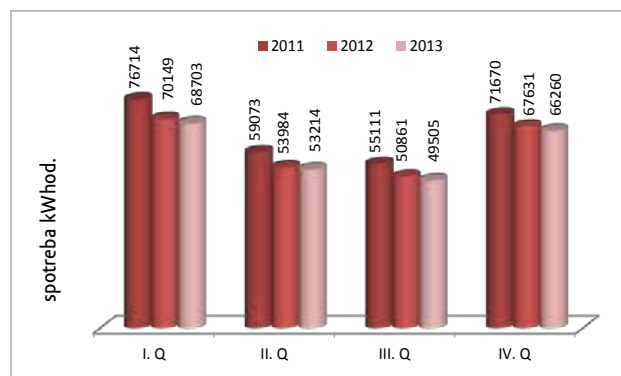
Graf č. 13: porovnanie spotreby elektrickej energie v hlavnej budove OLÚP, n.o. 2011–2013
