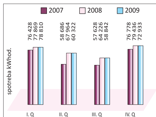
Graf č. 12: Porovnanie spotreby elektrickej energie v hlavnej budove OLÚP, n. o. 2007–2009
