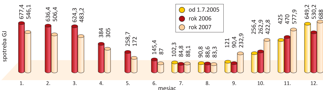
Graf č.1: Porovnanie spotreby tepla - hlavná budova
